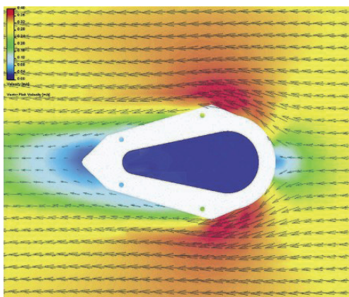
Διάγραμμα (CFD)
