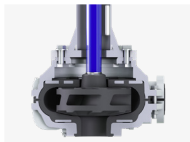
闭式叶轮 (橡胶衬里) 用于泥浆工况
