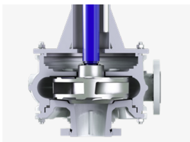
闭式叶轮用于泥浆工况
