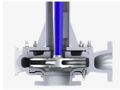
耐磨叶轮用于磨蚀性介质
